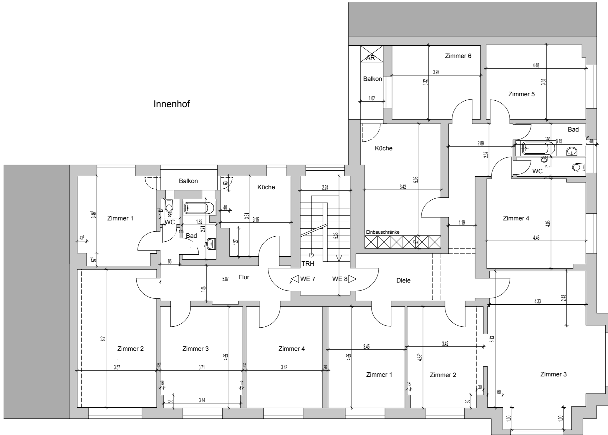
3.OG Bestand
