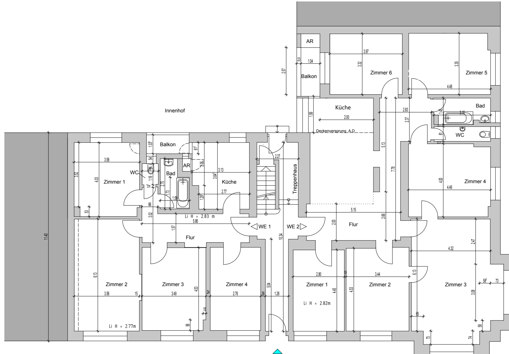
Grundriss EG Bestand
